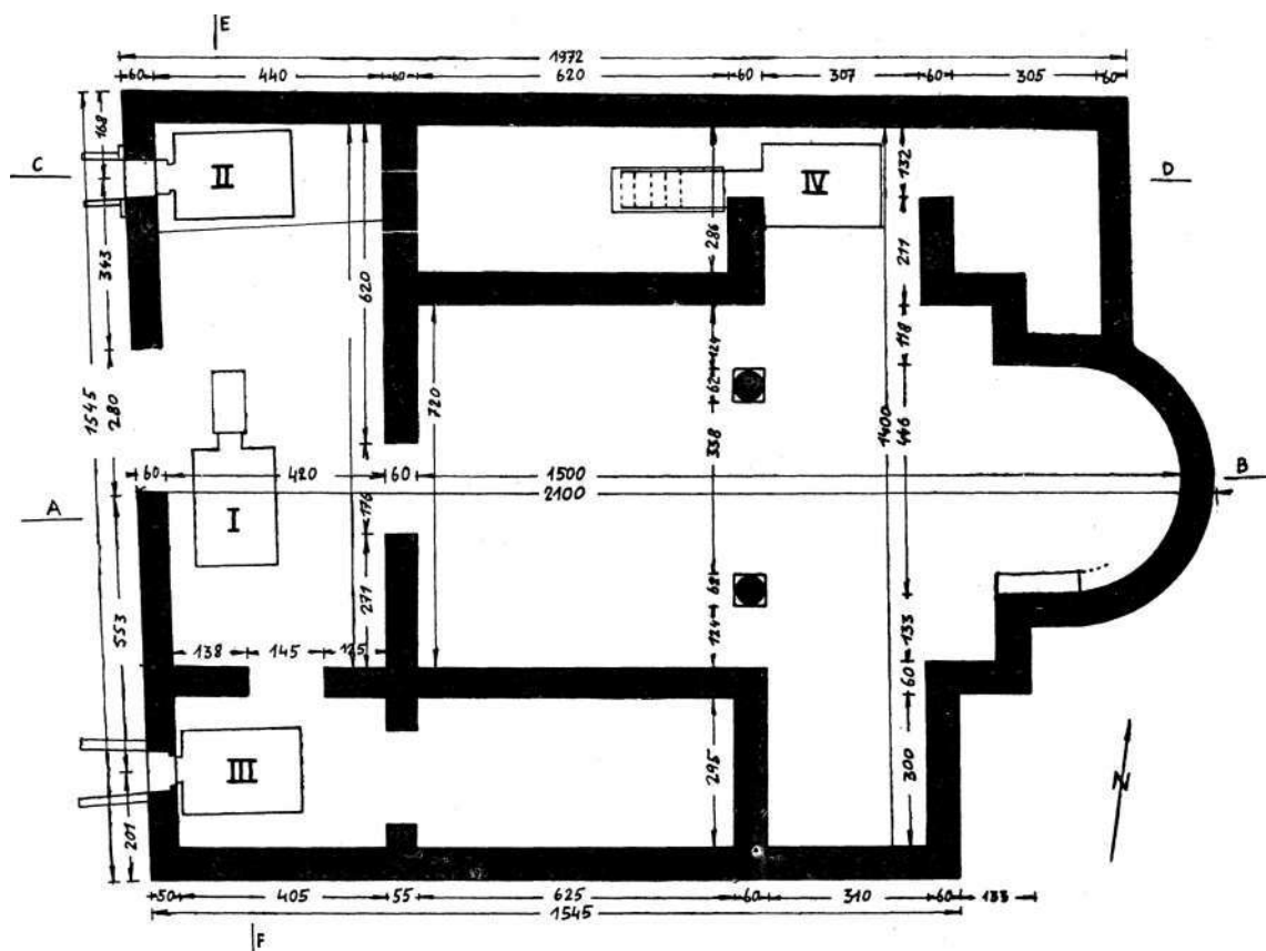
Sl. 3. Bazilika u Oborcima, tlocrt
