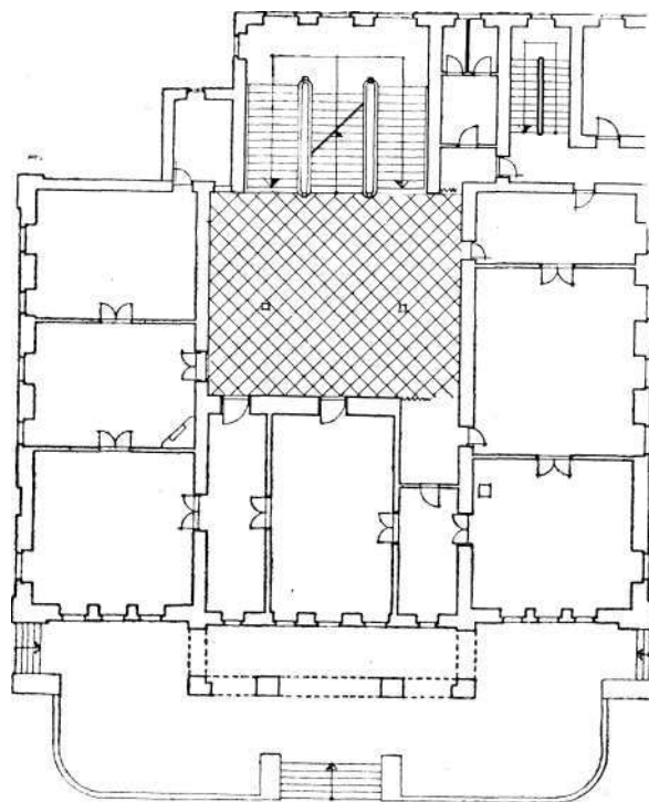
Sl. 9. i 10. Valijski konak u Sarajevu. Tlocrt prizemlja (gore), prvoga kata (dolje)
