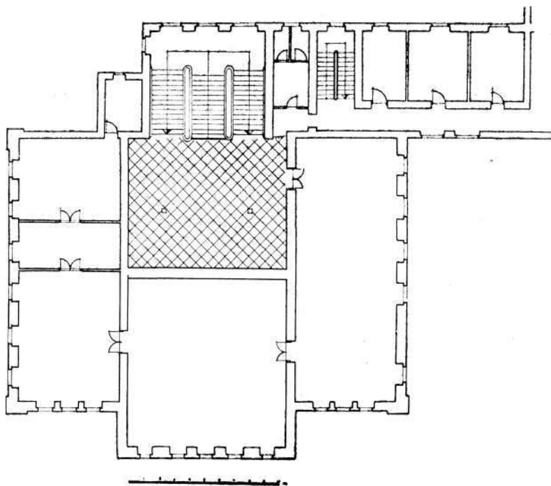
Sl. 11. Valijski konak u Sarajevu. Tlocrt drugoga kata.
