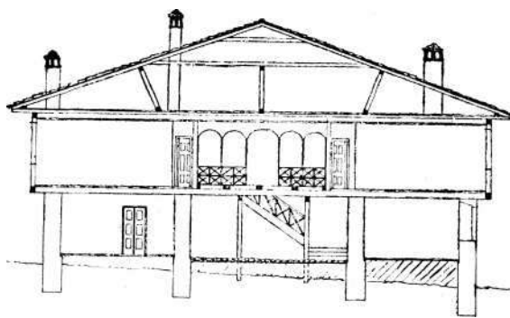
Sl. 1, 2 i 3. Valijki konak u Travniku. Tlocrt prizemlja (sredina) i ikata (gore) te poprečni presjek (dolje)
